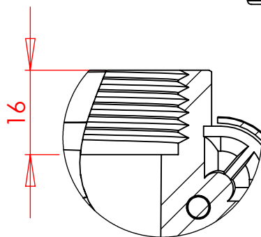
DETTAGLIO A SCALA 1 : 1
