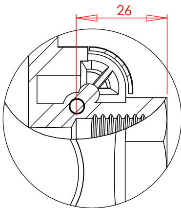
DETTAGLIO B SCALA 1 : 1
