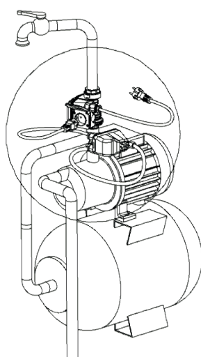
Utilizzo con gruppi di pressurizzazione o sistemi autoclave Use with pressurisation units or autoclave systems
